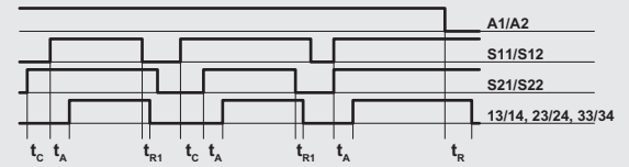
Konfiguration mit überwachtem Start
