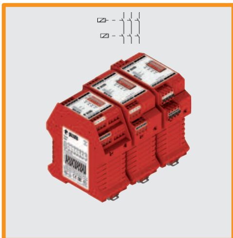
Erweiterungsmodul mit Ausgangskontakten, die bei Deaktivierung verzögert reagieren
