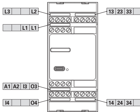
Anschlussbelegung CS AM22
