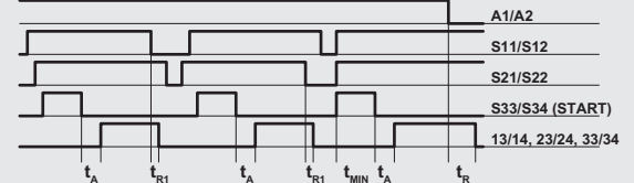
Konfiguration mit manuellem Start
