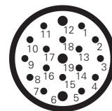
M23-Steckverbinder, 19-polig
