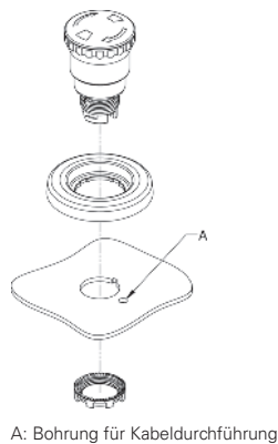
A: Bohrung für Kabeldurchführung
